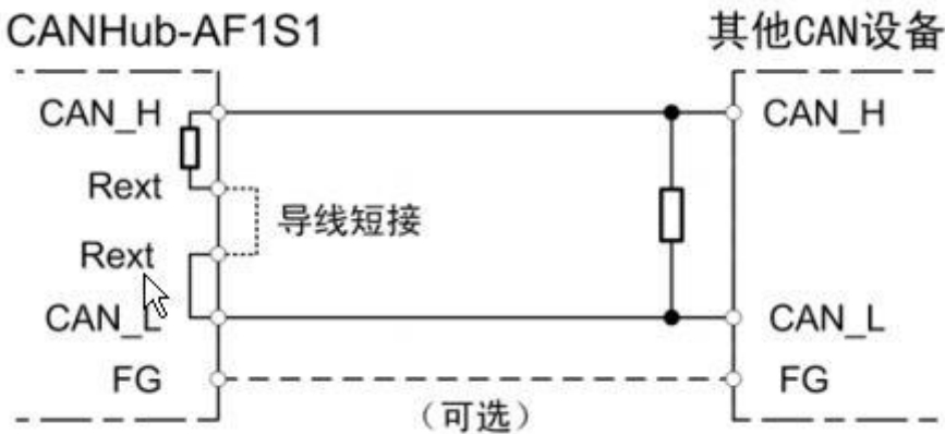
图 3.5 CANHub-AF1S1 通过双绞线接口连接于 CAN 网络
