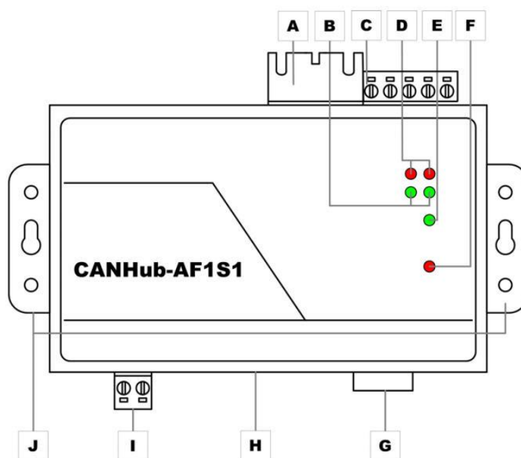
图 2.2 CANHub-AF1S1 各部件
