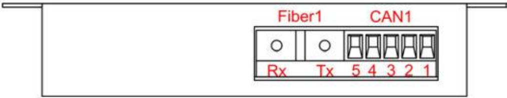
图 3.4 CANHub-AF1S1 通信接口
