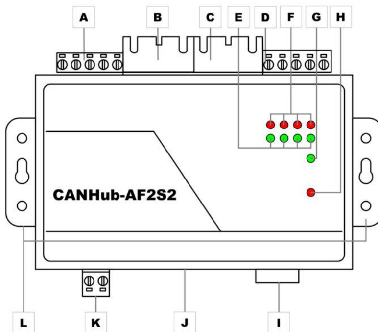
图 2.2 CANHub-AF2S2 各部件
