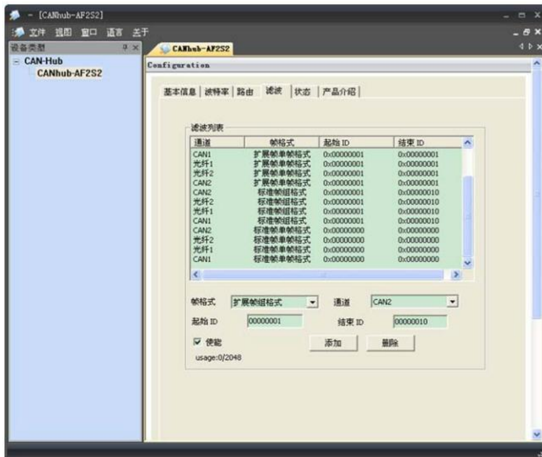
图 4.7 过滤功能
