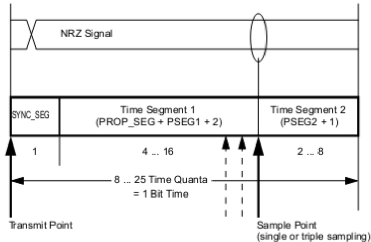
图 2.2 时间单位时序
